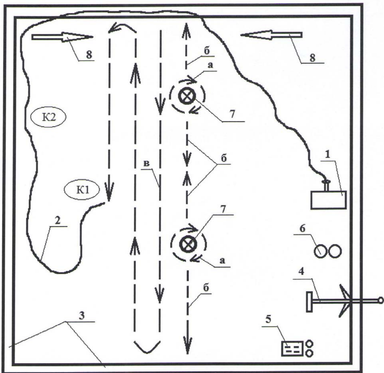
Рис.2. Схема организации рабочего места при устройстве кровли из жидкой резины «CBS кровельная», размещение установки непосредственно на крыше:
